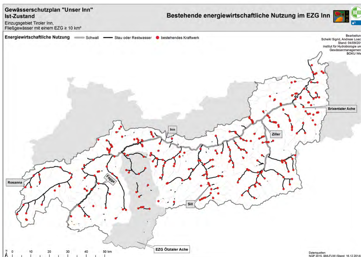
Abb. 6. Darstellung der bestehenden energiewirtschaftlichen Nutzung (Kraftwerke und genutzte Gewässerstrecken) im EZG Tiroler Inn
